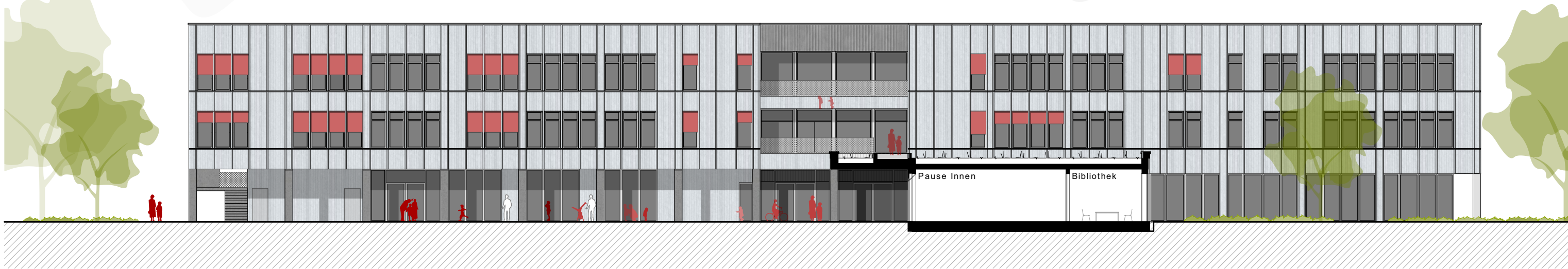
Ansicht Nord | M 1:250
