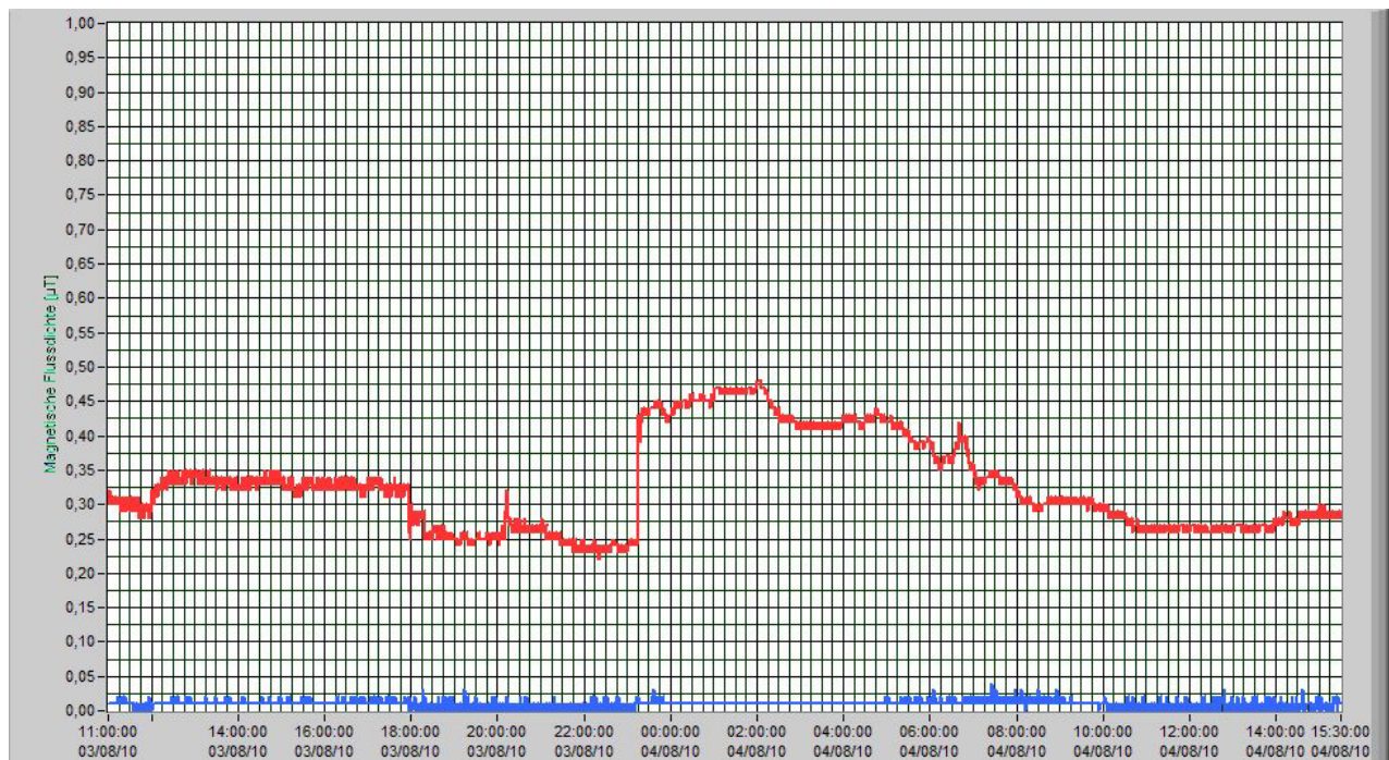
Abb. 8: Langzeitaufzeichnung am Referenzpunkt von Messlinie 1 (20 m); Aufzeichnungszeitraum 03.08.2010, 11:00 Uhr - 04.08.2010, 15:30 Uhr; vertikale Skalierung bis 1 \mu T
